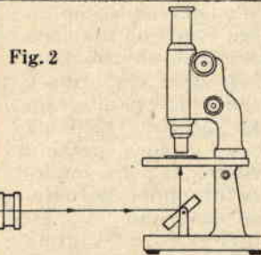
Fig. 2 - Per ingrandire l'immagine sopra lo schermo è necessario che il vetrino sia fortemente illuminato. Allo scopo può servire un piccolo proiettore che direzioni il fascio luminoso sullo specchietto.
