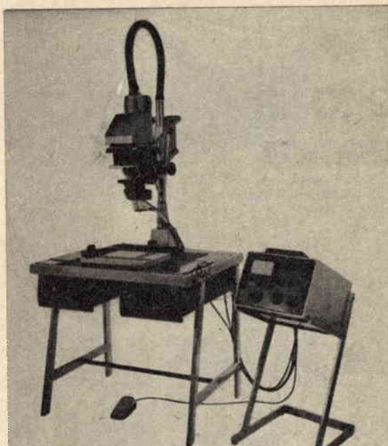
Ingranditore automatico Ferrania per il colore. Misura automaticamente le dominanti di colore e dà la giusta esposizione. È dotato di un vero cervello elettronico (a destra nella figura).
