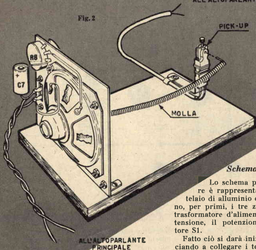
Fig. 2 - Il complesso costituito dall'altoparlante, dal pick-up e dalla molla deve essere montato a parte su una tavoletta di legno. Per i valori di C7 ed R8 vedi elenco componenti.
