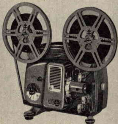
Nuovo proiettore per films 8 mm. della casa Pailard. Si distingue da tutti gli altri perchè può proiettare al rallentatore (velocità un terzo della normale) senza che l'immagine proiettata «balli». È dotato anche di retromarcia ed usa lampade da proiezione a basso voltaggio e minimo consumo. La bassa velocità di proiezione (5 fot/sec) è utilissima nei paesaggi e nelle vedute in genere che possono essere rimirate per molto tempo senza usare molta pellicola.
